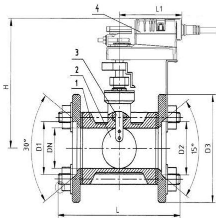
1 - корпус, 2 - диск, 3 - ось, 4 – ЭИМ
